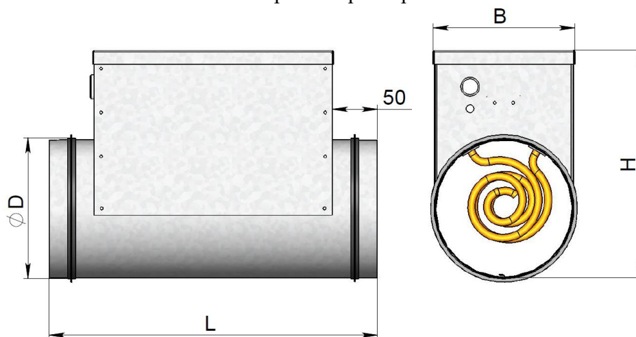
Габаритные размеры
